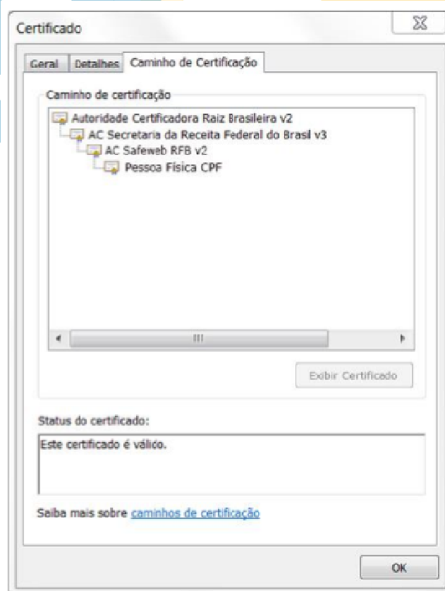
Imagem 02: Dados que compõem um CD
